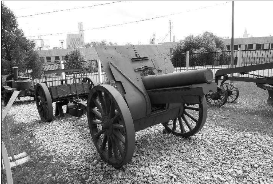
122-мм гаубица обр. 1910/30 гг. с передком в походном положении в экспозиции Центрального музея Великой Отечественной войны в г. Москве, вид спереди. Снимок автора.
