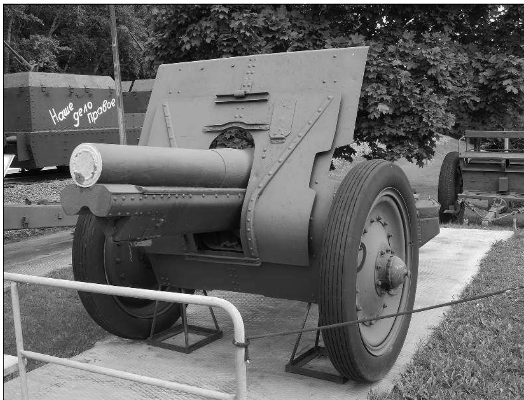
122-мм гаубица обр. 1910/30 гг. в экспозиции Центрального музея Великой Отечественной войны в г. Москве. Снимок автора.
