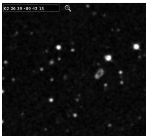
Объект 02 26 39–89 43 13 с интерактивной карты звёздного неба Sky-map.org: кольцевой объект — так называемый «Третий большой корабль»
