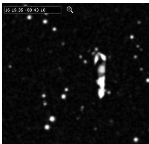
Объект 16 19 35–88 43 10 с интерактивной карты звёздного неба Sky-map.org: так называемый «Второй большой корабль»
