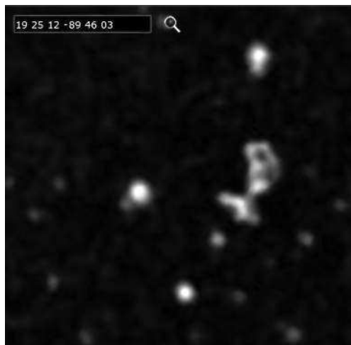
Объект 19 25 12–89 46 03 с интерактивной карты звездного неба Sky-map.org: так называемый «Первый большой корабль»
