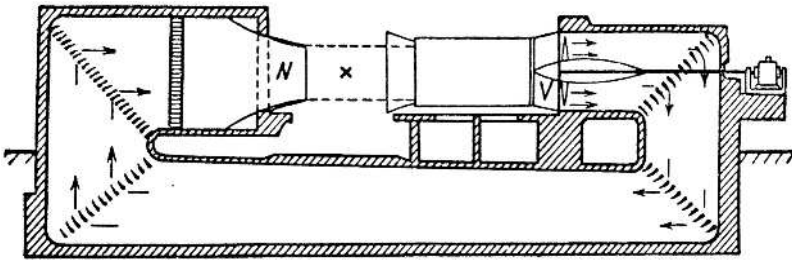
Рис. 3. Продольный разрез через аэродинамическую трубу. Модель крыла или самолета подвешивается в рабочем пространстве, отмеченном крестиком (x).
